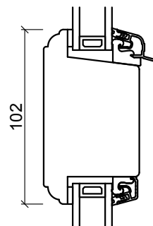
Senter Spennestykke
