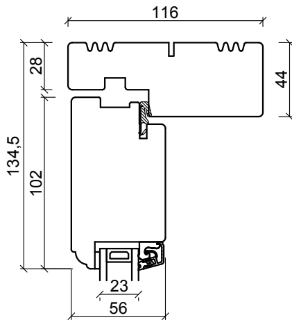
Toppkarm
