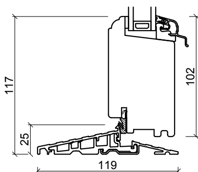
Bunnkarm (Alu-dørtrinn:)
