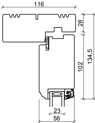
Toppkarm
