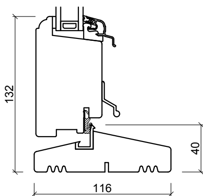
Bunnkarm
