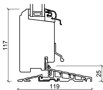
Bunnkarm (Alu-dørtrinn:)
