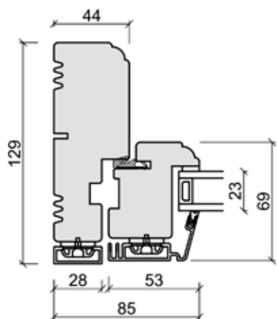
Sidekarm
