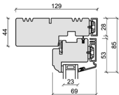
Tverpost - vannret
