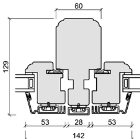
Mittpost, lodret
