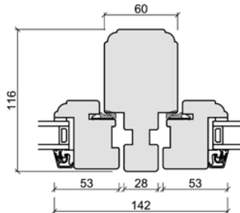
Mittpost, lodret
