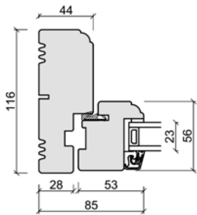
Sidekarm
