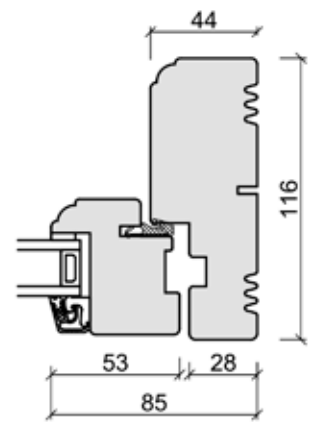
Sidekarm
