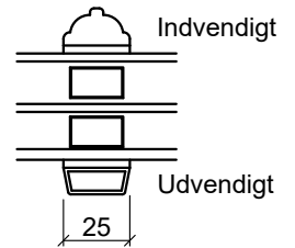
Energisprosse
