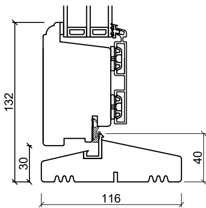
Hårdtræs Bundkarm
