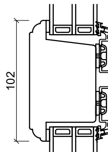
Spændestykke
