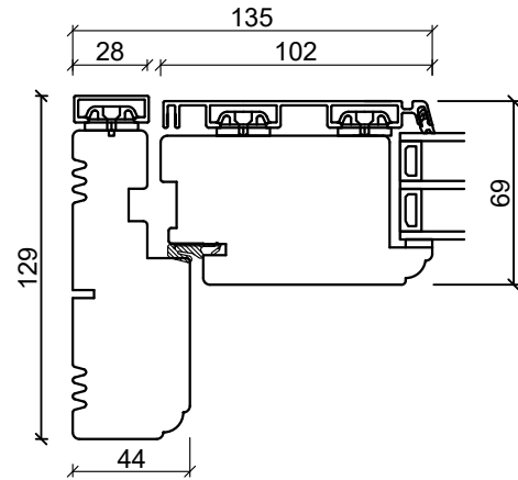
Sidekarm
