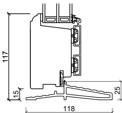
Glasfiber Bundkarm
