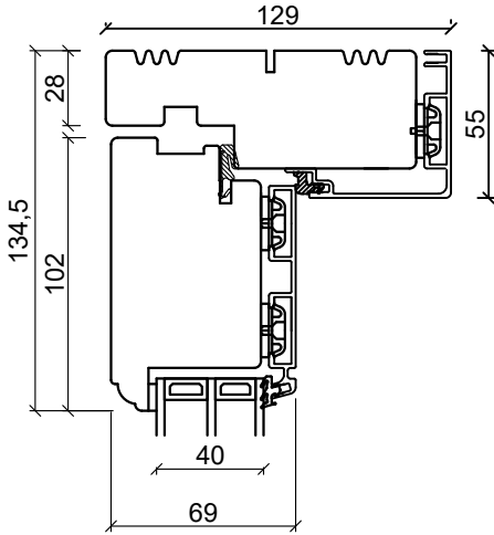
Overkarm
