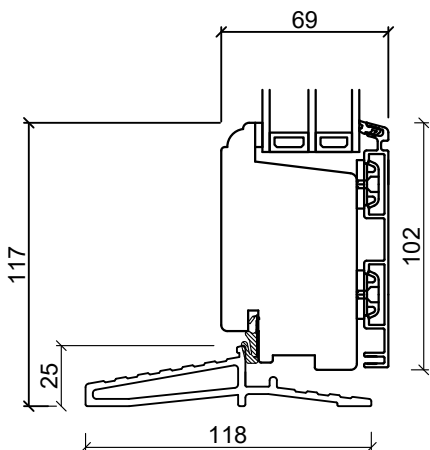
Glasfiber Bundkarm
