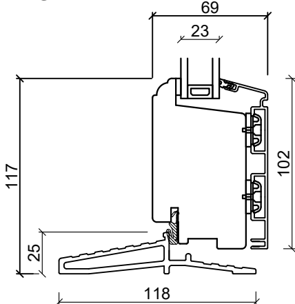
Glassfiber Bunnkarm
