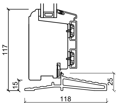
Glassfiber Bunnkarm
