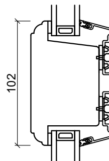
Spennstykke
