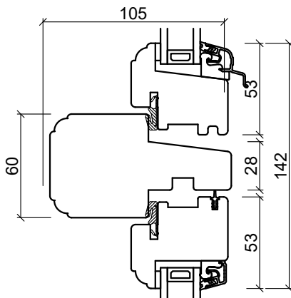
Tverpost, vannret
