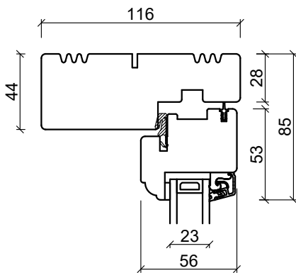
Toppkarm
