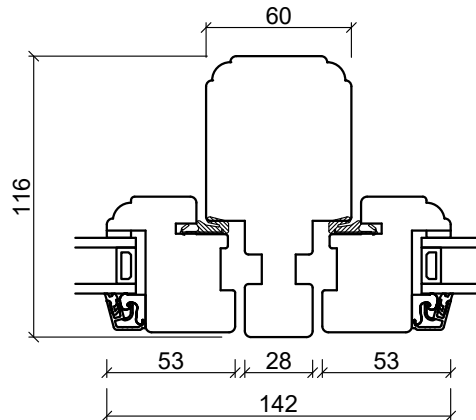
Mittpost, lodret
