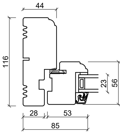
Sidekarm
