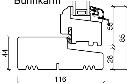
Bunnkarm
