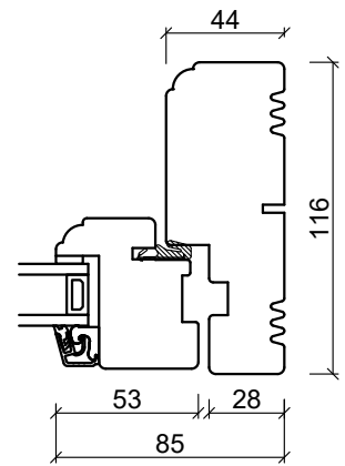
Sidekarm
