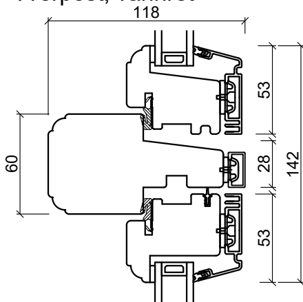
Tverpost, vannret
