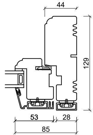
Sidekarm
