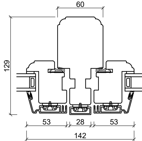
Mittpost, lodret
