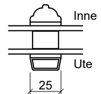
Energisprosse
