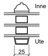
Energisprosse
