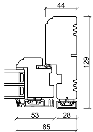
Sidekarm
