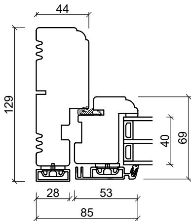
Sidekarm
