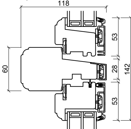
Tverpost, vannret
