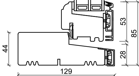
Bunnkarm
