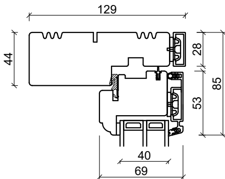
Toppkarm
