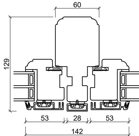
Mittpost, lodret
