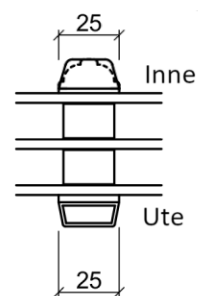
Energisprosse
