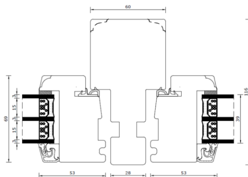
Mittpost, lodret
