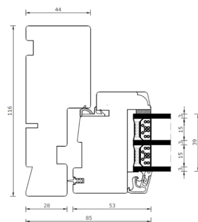
Sidekarm
