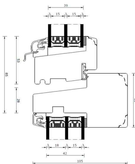
Tverpost, vannret
