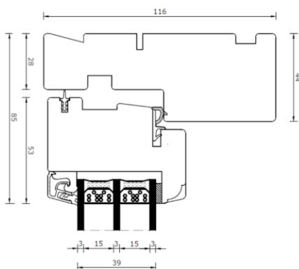
Toppkarm
