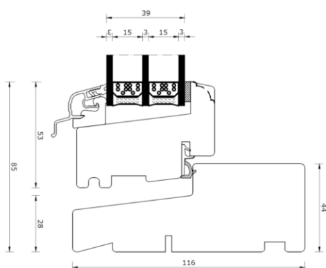
Bunnkarm
