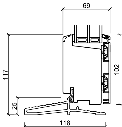
Glassfiber Bunnkarm
