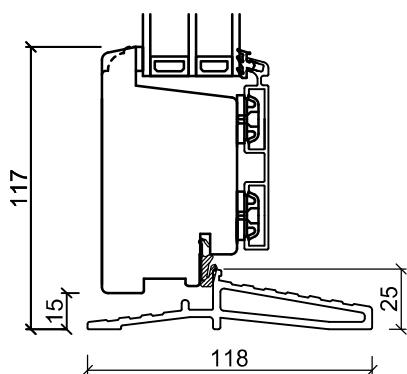
Glassfiber Bunnkarm
