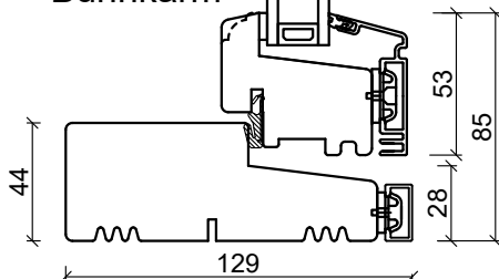
Bunnkarm
