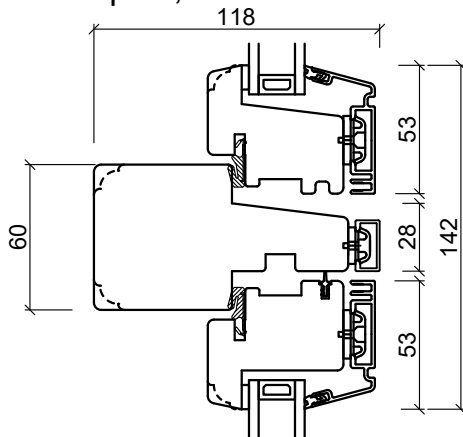
Tverpost, vannret
