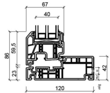
Bunnkarm
