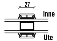
Sprosse
