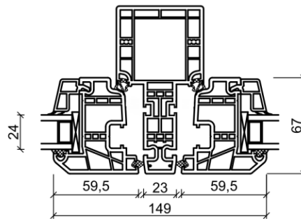
Mittpost, lodret
