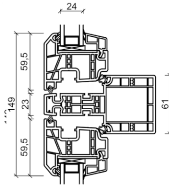
Tverpost, lodret
