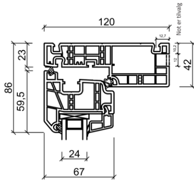
Toppkarm
