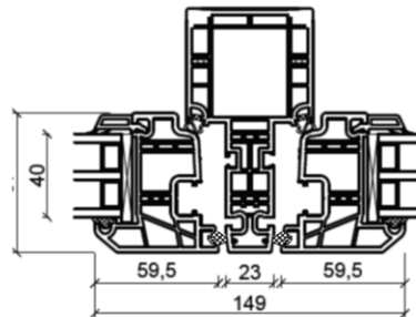
Mittpost, lodret
