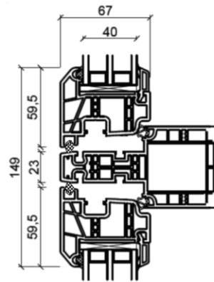
Mittpost, lodret
