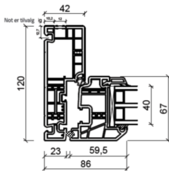
Sidekarm
