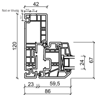
Sidekarm
