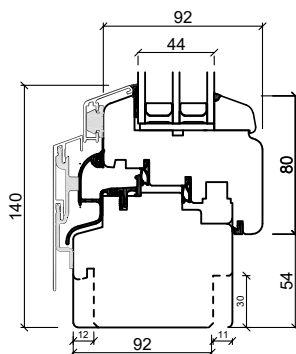
Bunnkarm
