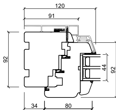
Tre bunnkarm
