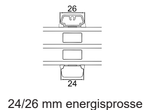
Energisprosse
