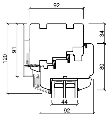
Midt dobbeldør
