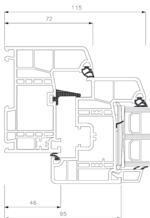
Sidekarm
