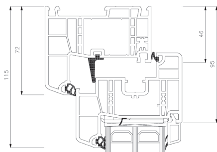
Overkarm
