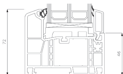
Bunnkarm
