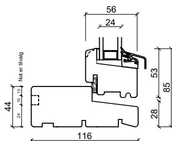
Bunnkarm
