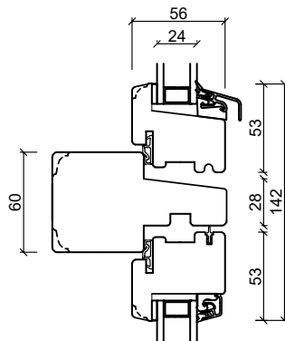
Tverrpost – vannrett
