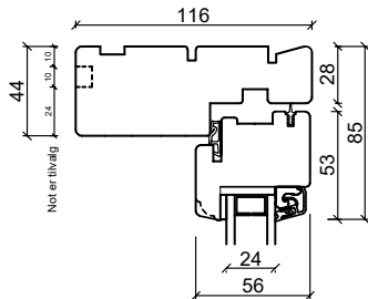
Overkarm
