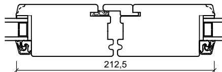
Midt dobbeldør
