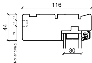
Overkarm
