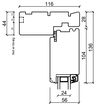
Overkarm
