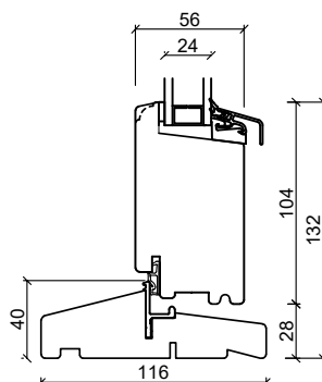
Hardtre dørterskel
