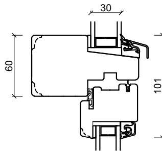
Tverrrpost
