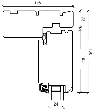
Vannrett post
