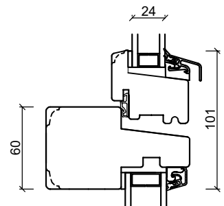
Tverrrpost
