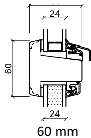
Vannrett post
