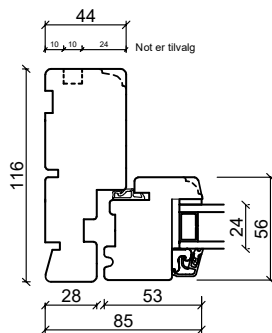
Sidekarm
