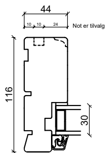
Sidekarm
