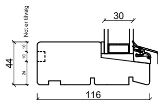
Bunnkarm
