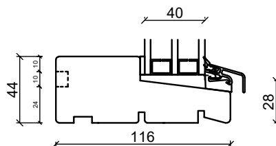
Bunnkarm
