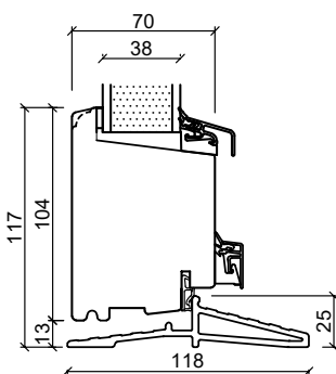
Fiber dørterskel
