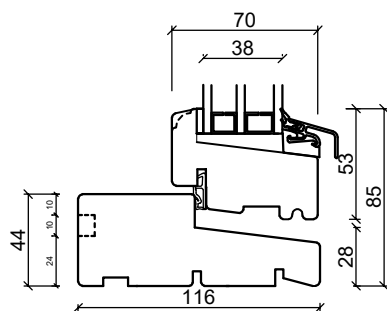
Bunnkarm
