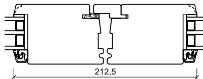
Midt dobbeldør
