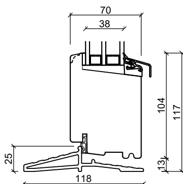
Fiber dørterskel
