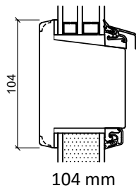
Fiber dørterskel
