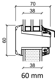
Vannrett post
