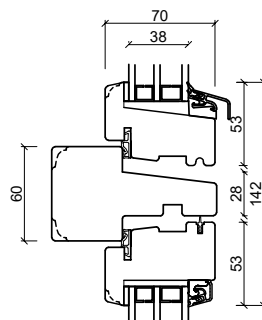
Tverrpost – vannrett
