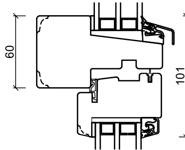
Tverrrpost
