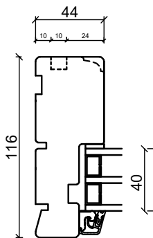
Sidekarm
