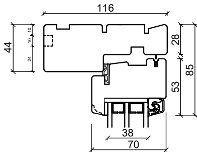
Overkarm
