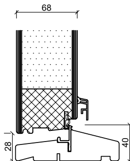
Hardtre dørterskel
