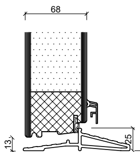
Fiber dørterskel
