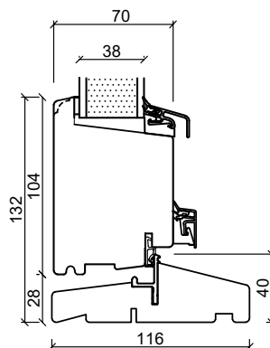
Hardtre dørterskel
