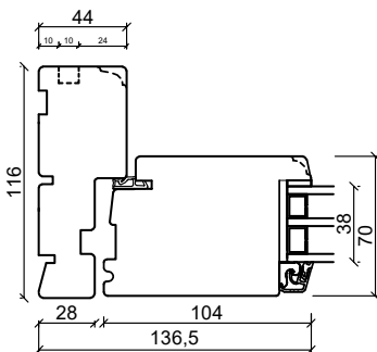
Sidekarm
