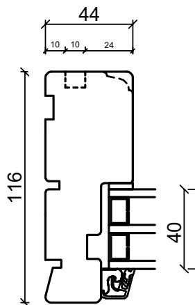
Bunnkarm
