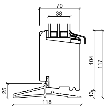
Fiber dørterskel
