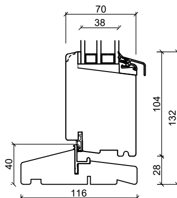
Hardtre dørterskel
