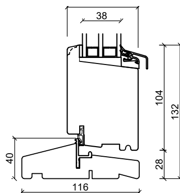
Hardtre dørterskel
