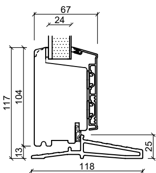
Fiber dørterskel
