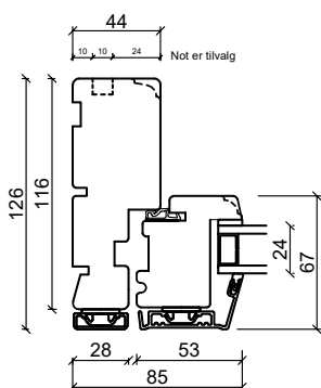
Sidekarm
