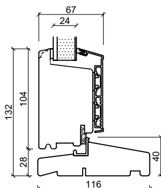
Hardtre dørterskel
