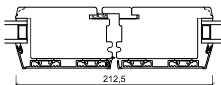
Midt dobbeldør
