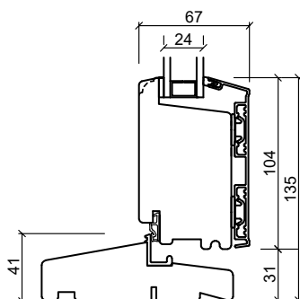
Hardtre dørterskel
