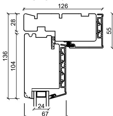
Overkarm
