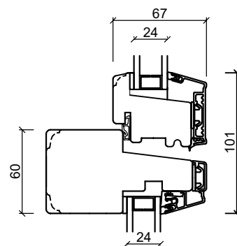
Tverrrpost
