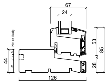
Bunnkarm
