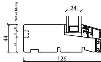
Bunnkarm
