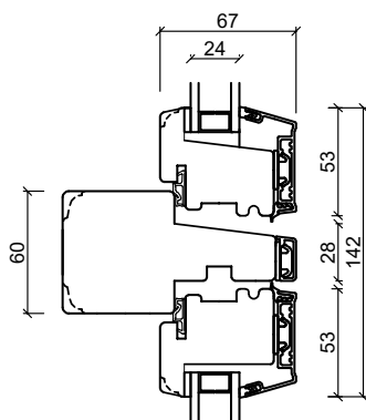
Tverrpost – vannrett
