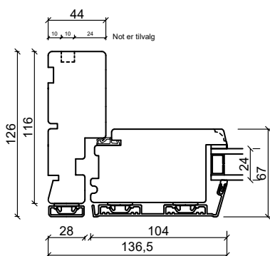
Sidekarm
