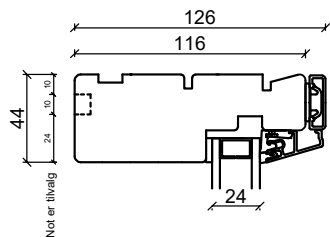
Overkarm
