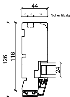
Sidekarm
