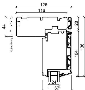
Overkarm
