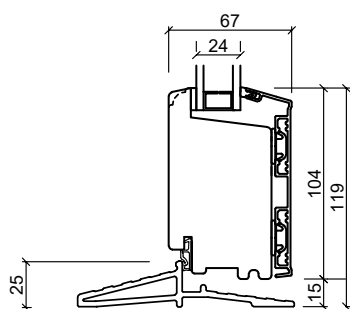
Fiber dørterskel
