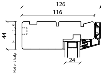
Overkarm
