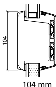
Fiber dørterskel
