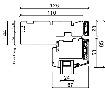
Overkarm
