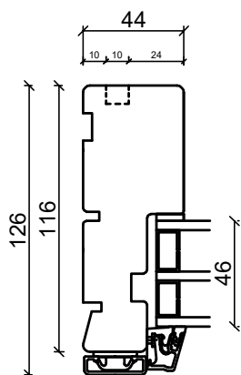
Sidekarm
