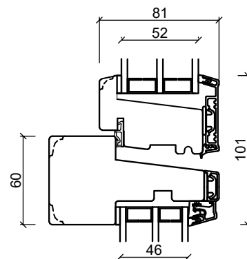
Tverrrpost
