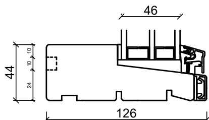
Bunnkarm
