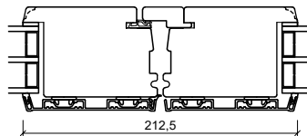
Midt dobbeldør
