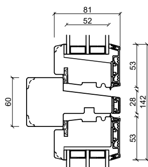
Tverrpost – vannrett
