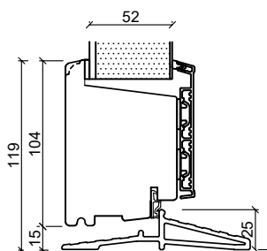
Fiber dørterskel
