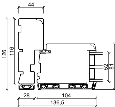
Fiber dørterskel
