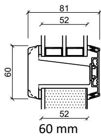
Vannrett post
