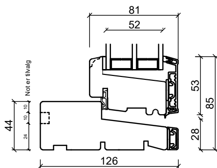
Bunnkarm
