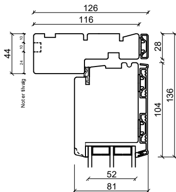
Overkarm
