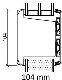
Fiber dørterskel
