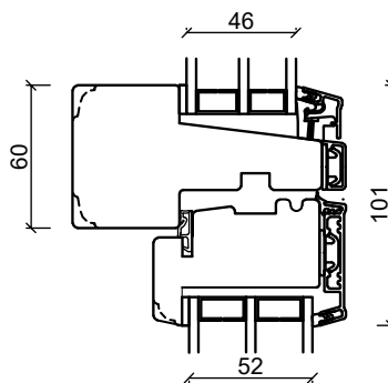
Tverrrpost
