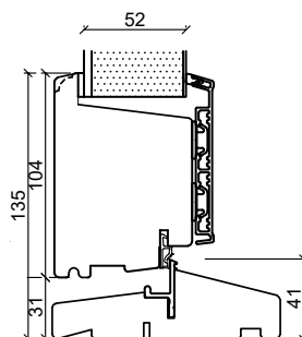
Hardtre dørterskel
