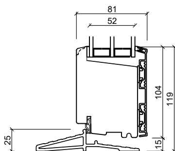
Fiber dørterskel
