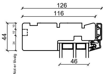
Sidekarm
