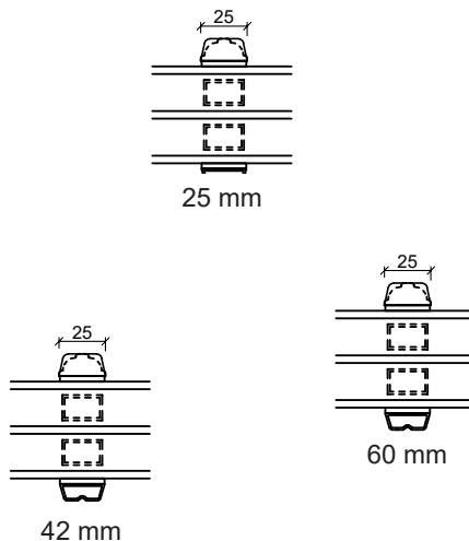
Energisprosse
