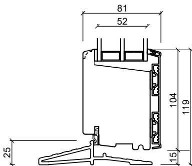
Fiber dørterskel
